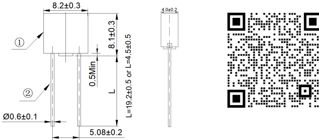
6-1 工程圖 ( 單位 : mm ) / Outline Drawing and Dimensions (Unit: mm)
